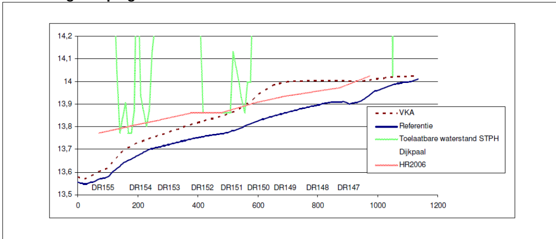
Afbeelding 2. Piping
