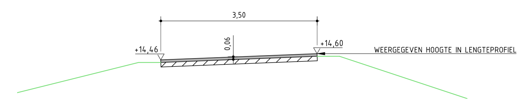
PRINCIPE DOORSNEDE A-A SCHAAL 1:50
